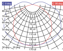
Кривые силы света
