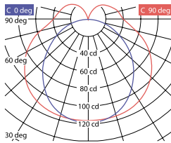
Кривые силы света
